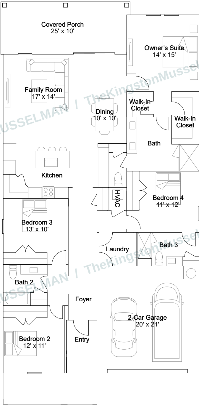
Elevation E5
